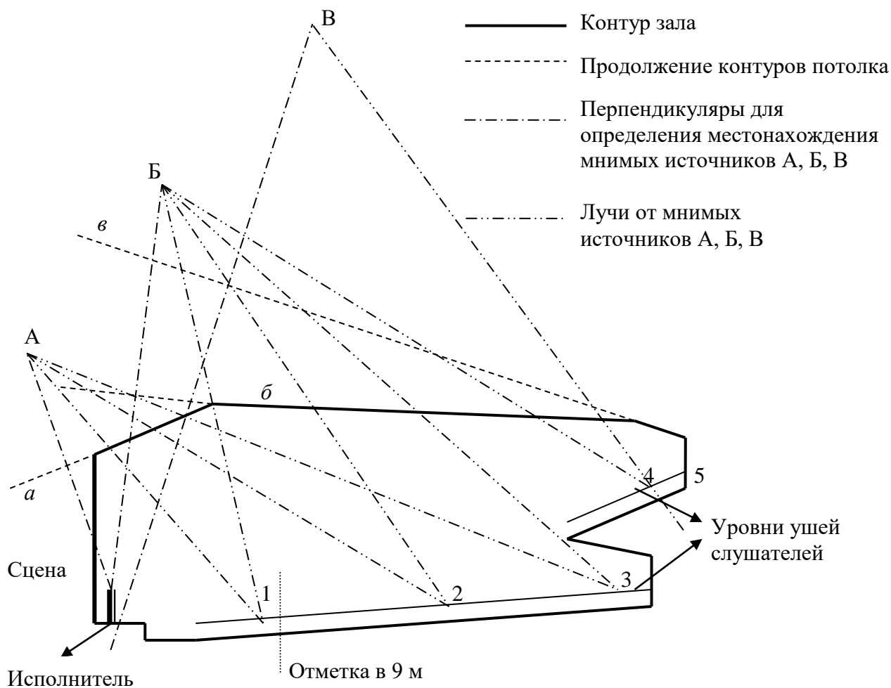
Рисунок 1.22 – Разрез зала с лучевым эскизом
