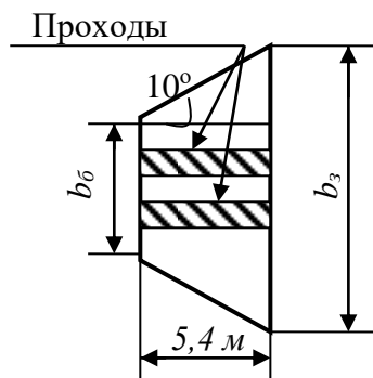
Рисунок 1.21 – Схематическое изображение плана балкона
