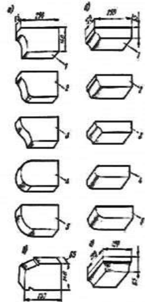
ЛЕКАЛЬНЫЙ КИРПИЧ
