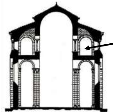
ЭМПОРЫ
