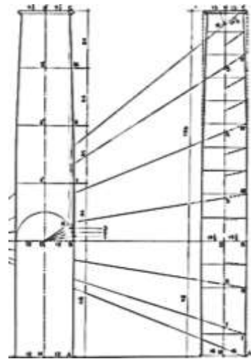
ЭНТАЗИС
