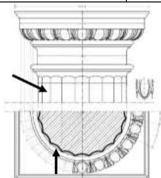
КАННЕЛЮРЫ
