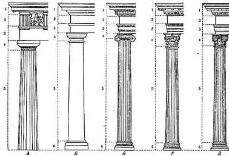
ОРДЕР
