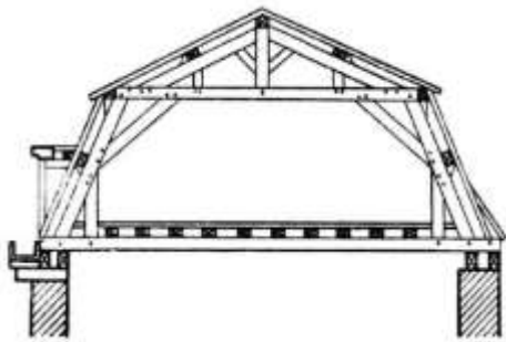
МАНСАРДА
