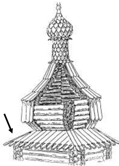
УСЕЧЕННАЯ ПИКА
