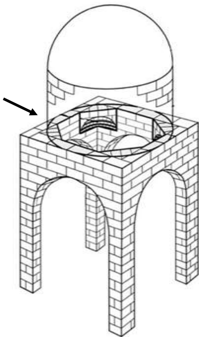
ТРОМП
