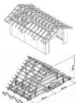
СТРОПИЛА
