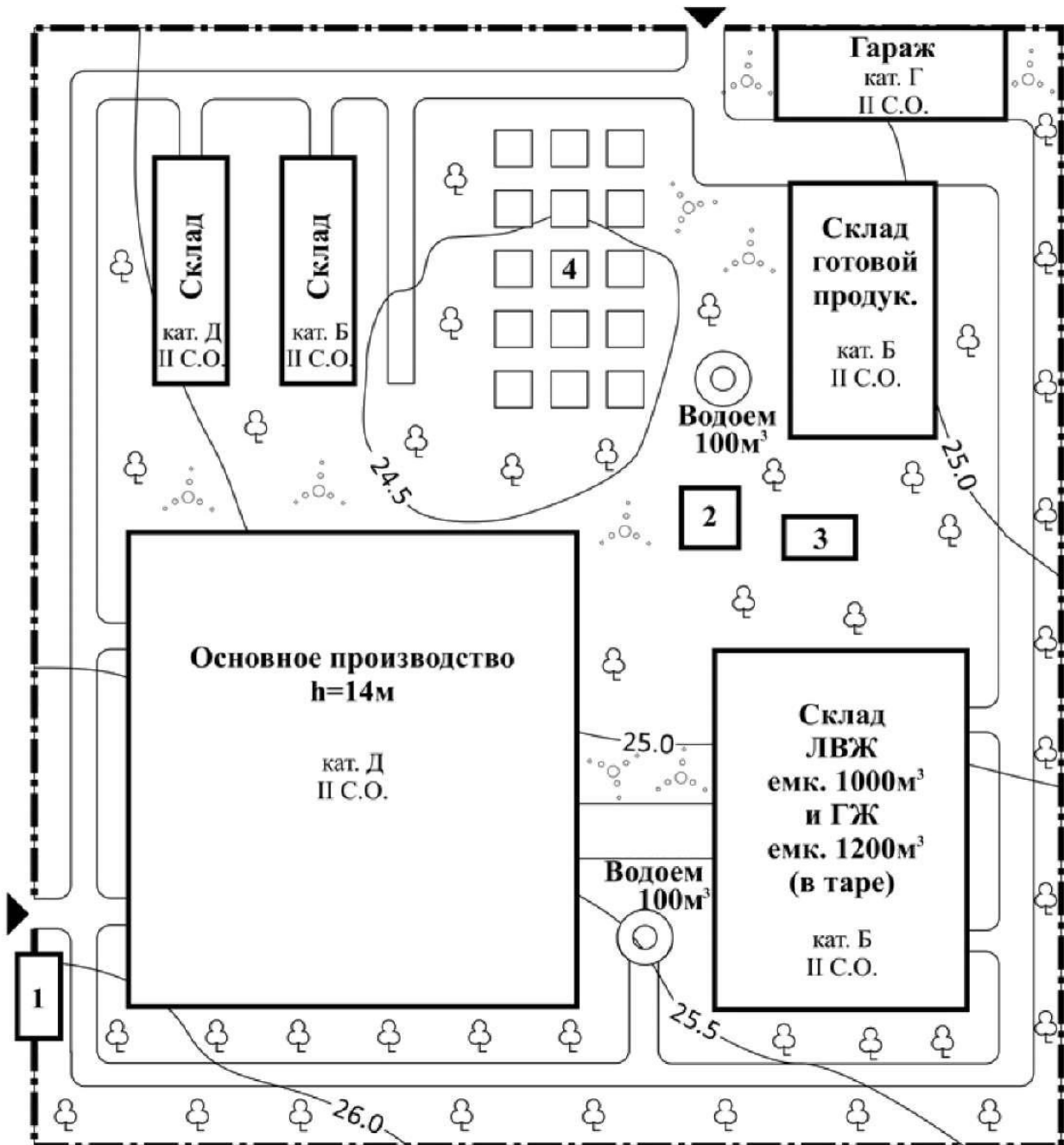
1 – контрольно-пропускной пункт, II С.О.; 2 – трансформаторная подстанция, II С.О.; 3 – насосная, II С.О.; 4 – склад леса, ёмк. 6000 м
