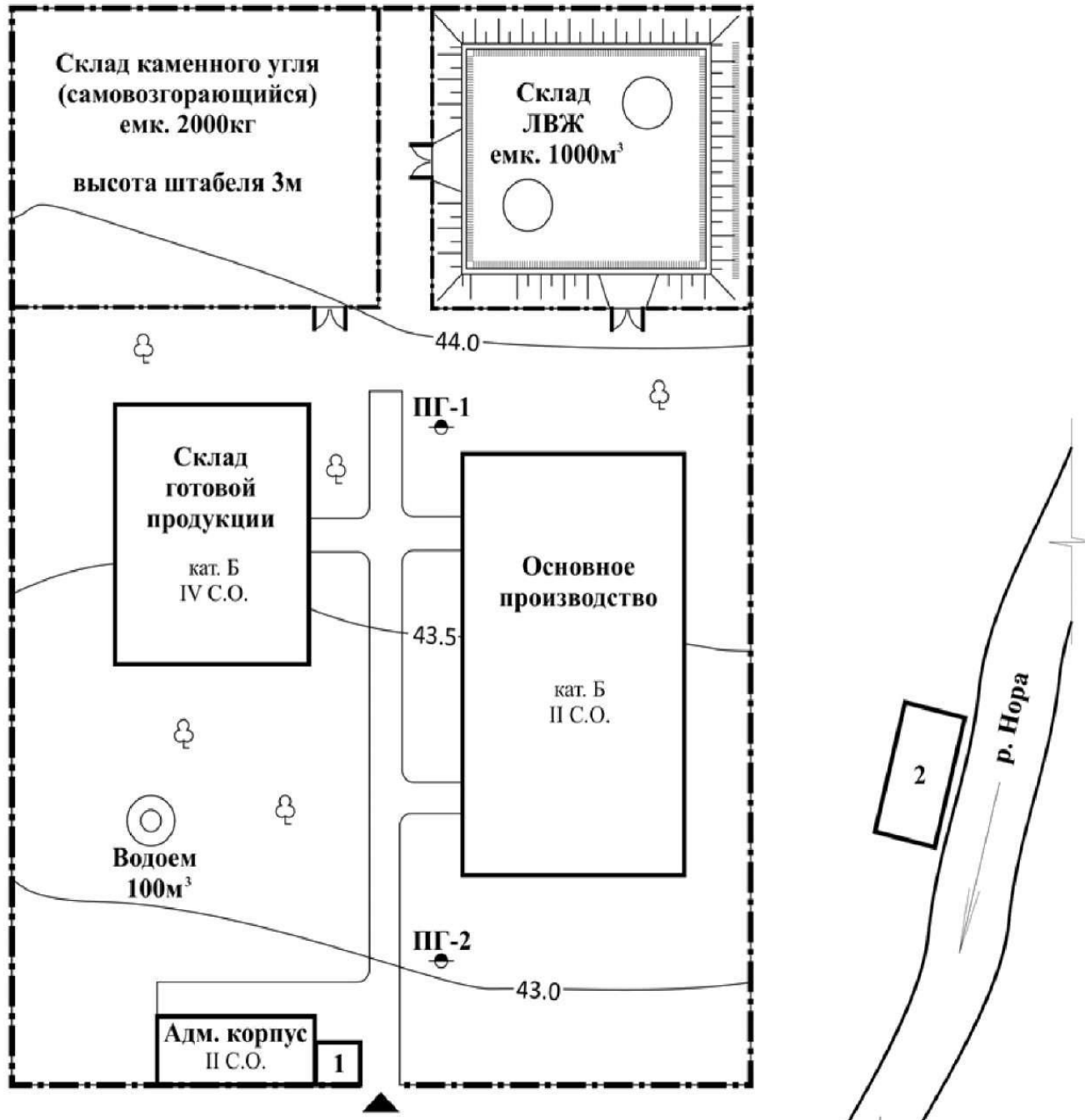
1 – контрольно-пропускной пункт, II С.О.; 2 – речной док Рисунок А.4 – Генеральный план предприятия
