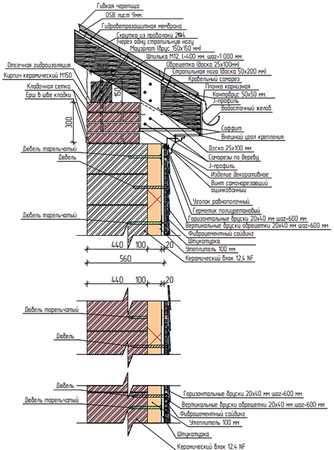
Рисунок 40 – Вариантное решение разреза по стене
