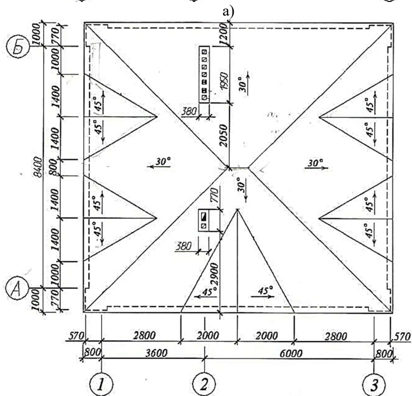
Рисунок 28 – Пример выполнения практической работы № 5. Схема стопил
