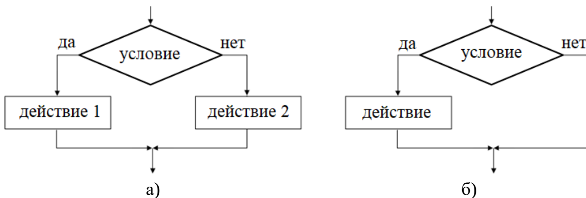
Рисунок 3 – Блок-схема ветвящегося процесса
