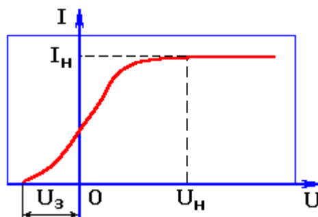
Рисунок 3 – Вольтамперная характеристика внешнего фотоэффекта
