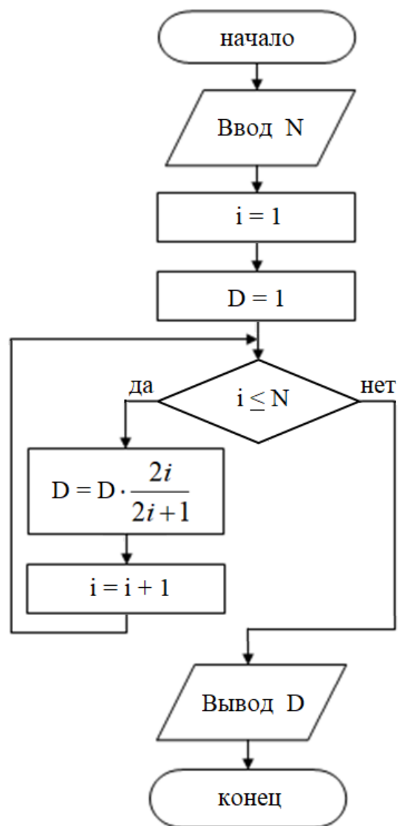
а – блок-схема алгоритма к примеру 16; б – блок-схема алгоритма к примеру 17 Рисунок 21 – Блок-схемы к примерам 16 и 17
