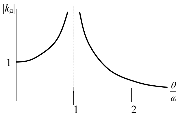
Рисунок 20.8 - График k_d\left(\frac{\theta}{\omega}\right)
