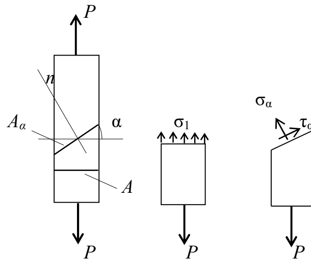
Рисунок 16.4 – Линейное напряженное состояние
