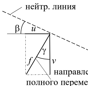
Рисунок 18.9 – Перемещения при косом изгибе
