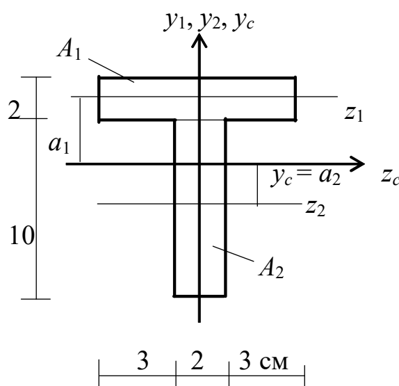
Рисунок 13.11 – Тавровое сечение
