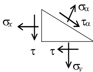
Рисунок 17.1 – Напряжения по наклонной площадке
