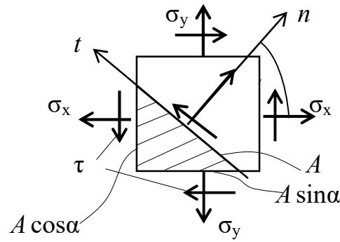
Рисунок 16.7 – Плоское напряженное состояние
