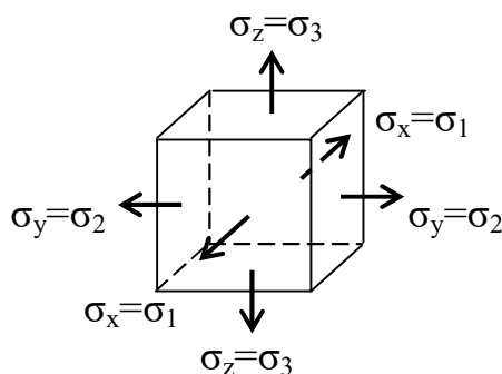
Рисунок 16.3 – Трехосное напряженное состояние
