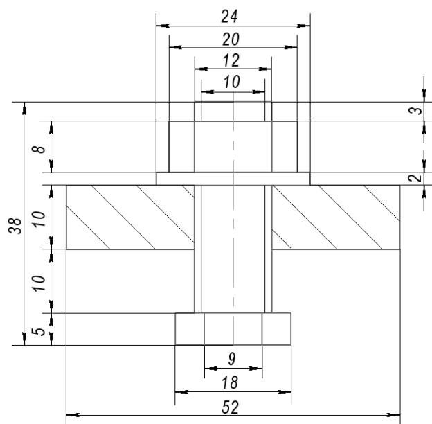
Рисунок 43 – Исходные данные для выполнения чертежа болтового соединения
