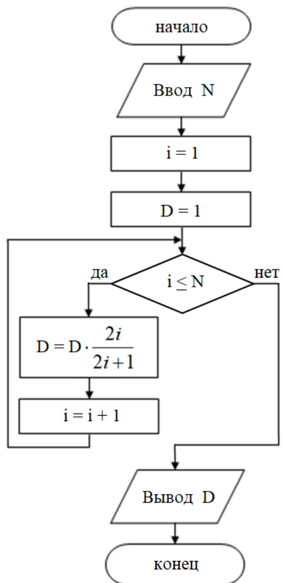
Рисунок 21 – Блок-схемы к примерам 16 и 17
