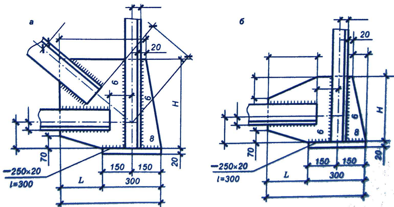
а) с раскосом
