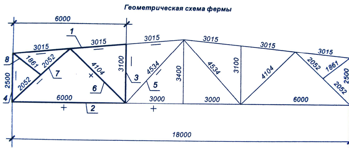
Рисунок 5.1 – Пример выполнения геометрической схемы фермы
