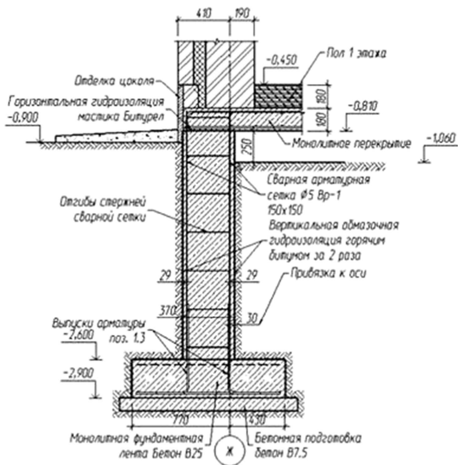
Рисунок 36 – Вариантные решения сборного ленточного фундамента под наружную кирпичную стену
