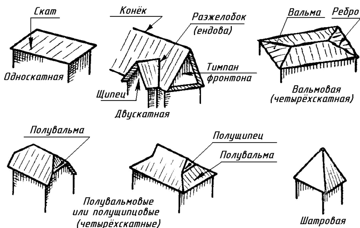
Рисунок 2.5 – Типы крыш
