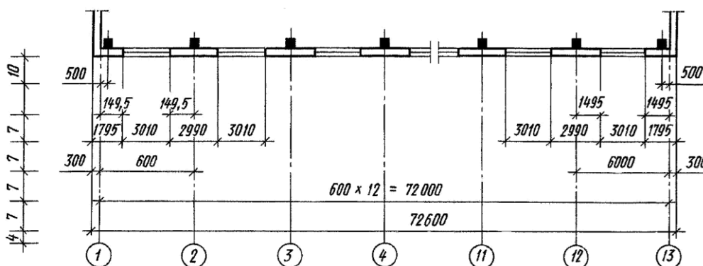
При наличии в изображении ряда одинаковых элементов, расположенных на равных расстояниях друг от друга, размеры между ними проставляют только в начале и в конце ряда и указывают суммарный размер между крайними элементами в виде произведения числа повторений на повторяющийся размер.
