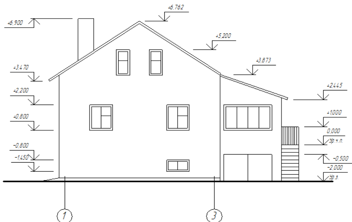
Рисунок Г.1 – Пример выполнения чертежа фасада
