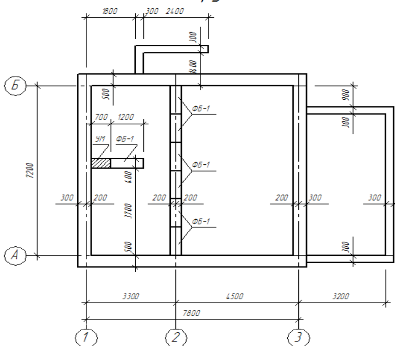
План фундаментов
