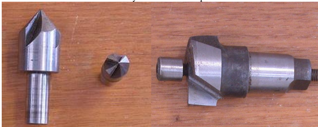
Рисунок 3.20 – Зенковка (слева) и цековка (справа)
