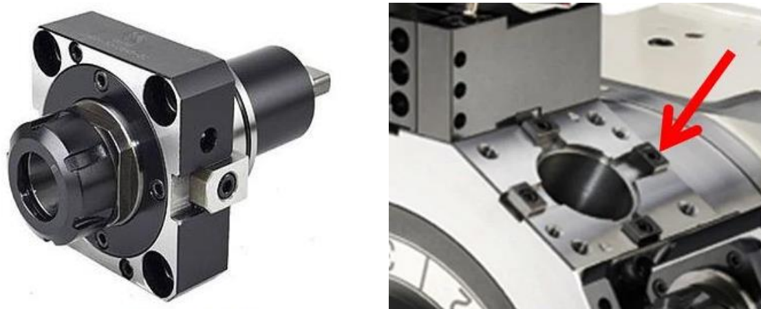
Рисунок 5.6 – Инструментальный блок с системой крепления BMT
