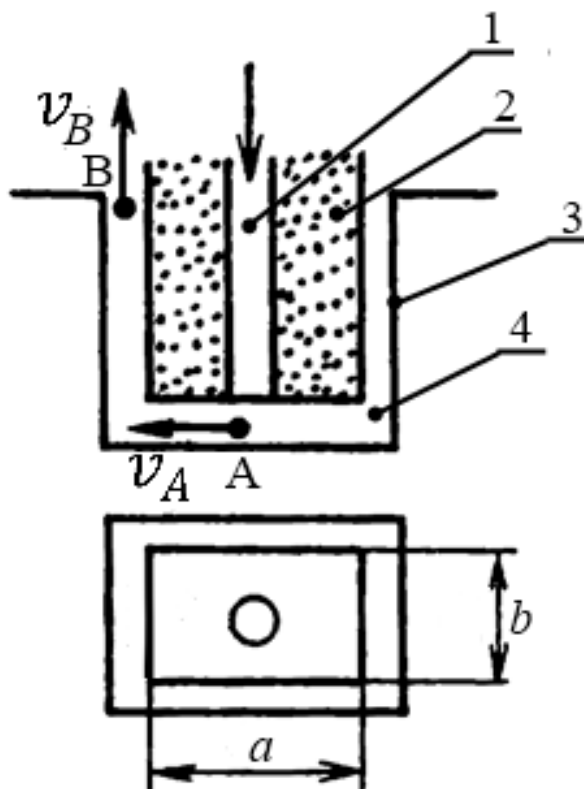
Рисунок 1.1 – Обработка прямоугольной призматической полости
