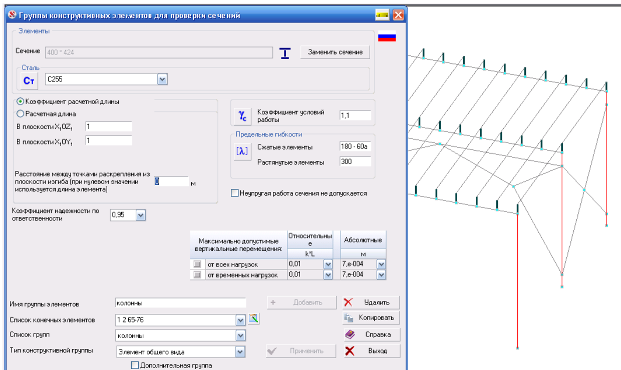
Рисунок 2.14 – Назначение группы «Колонны»
