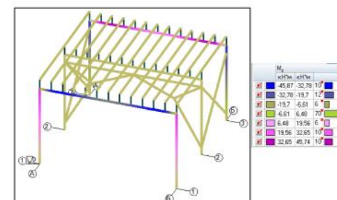
Эпюры моментов M_z
