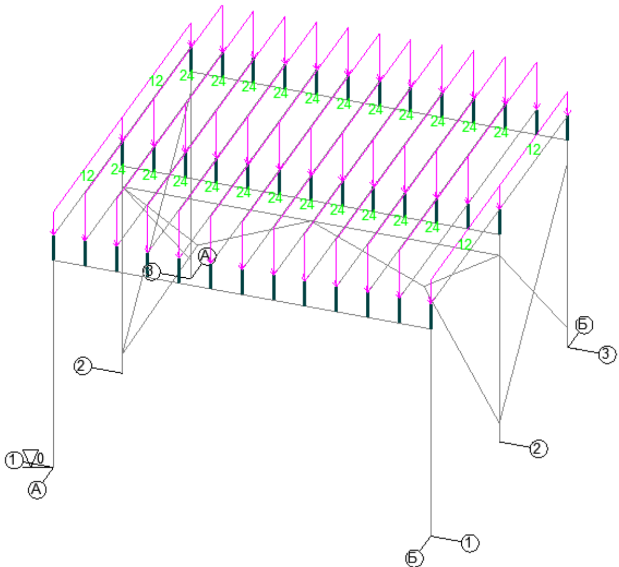
Рисунок 2.4 – Временная нагрузка на второстепенные балки
