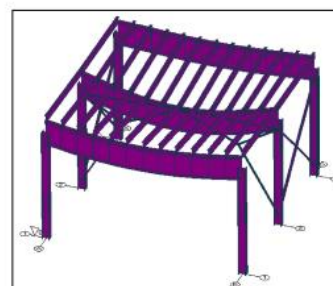
Деформированная схема
