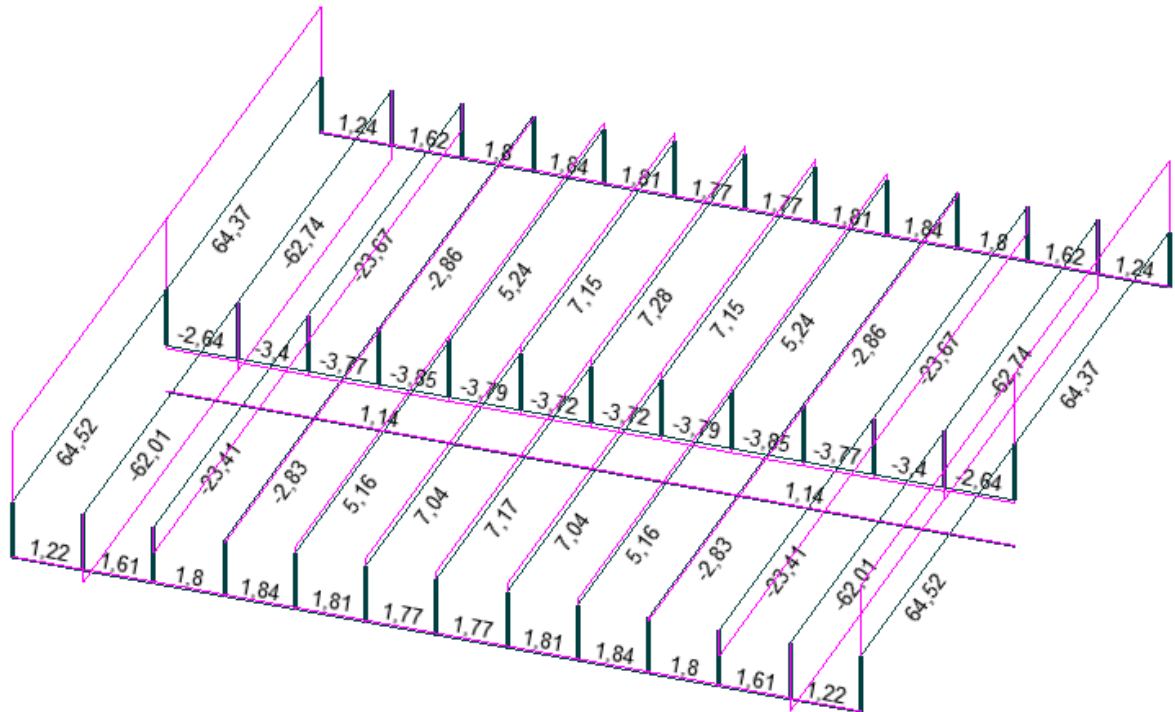
Рисунок 2.5 – Балки перекрытия. Эпюры усилий N
