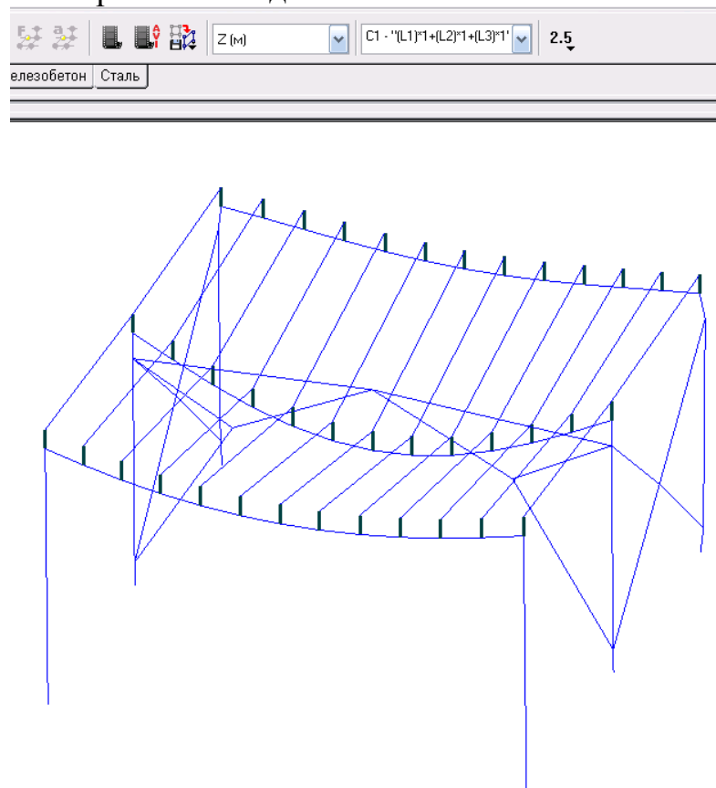
Рисунок 2.18 – Деформированная схема
