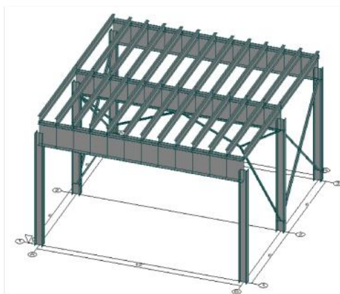
Расчетная схема балочной клетки
