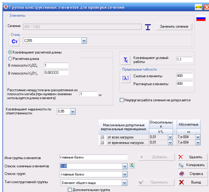
Рисунок 2.12 – Назначение группы – «Главные балки»
