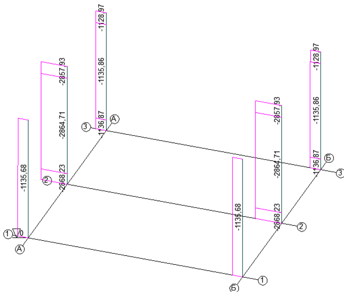
Рисунок 2.8 – Эпюры усилий N . Колонны
