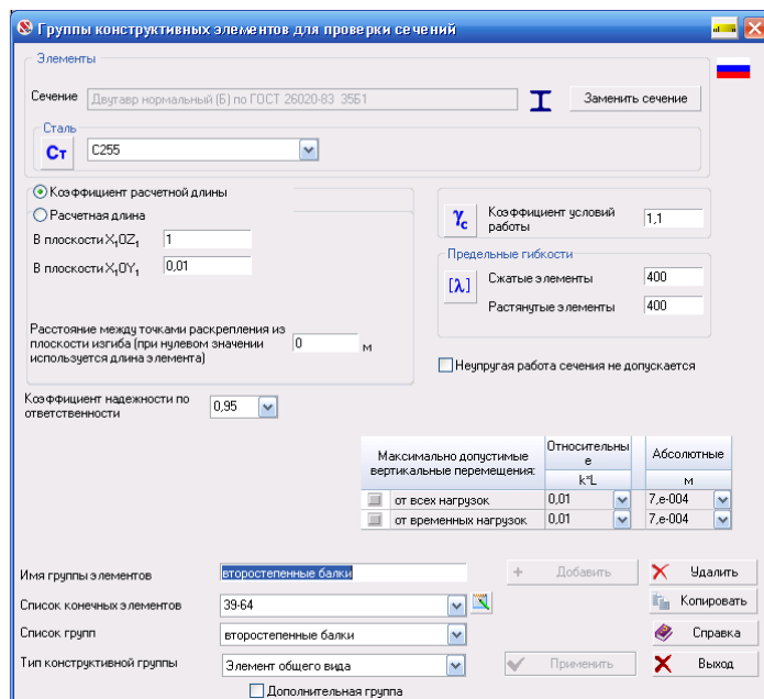
Рисунок 2.13 – Назначение группы – «Второстепенные балки»
