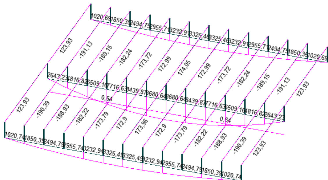
Рисунок 2.6 – Балки перекрытия. Эпюры усилий M_y
