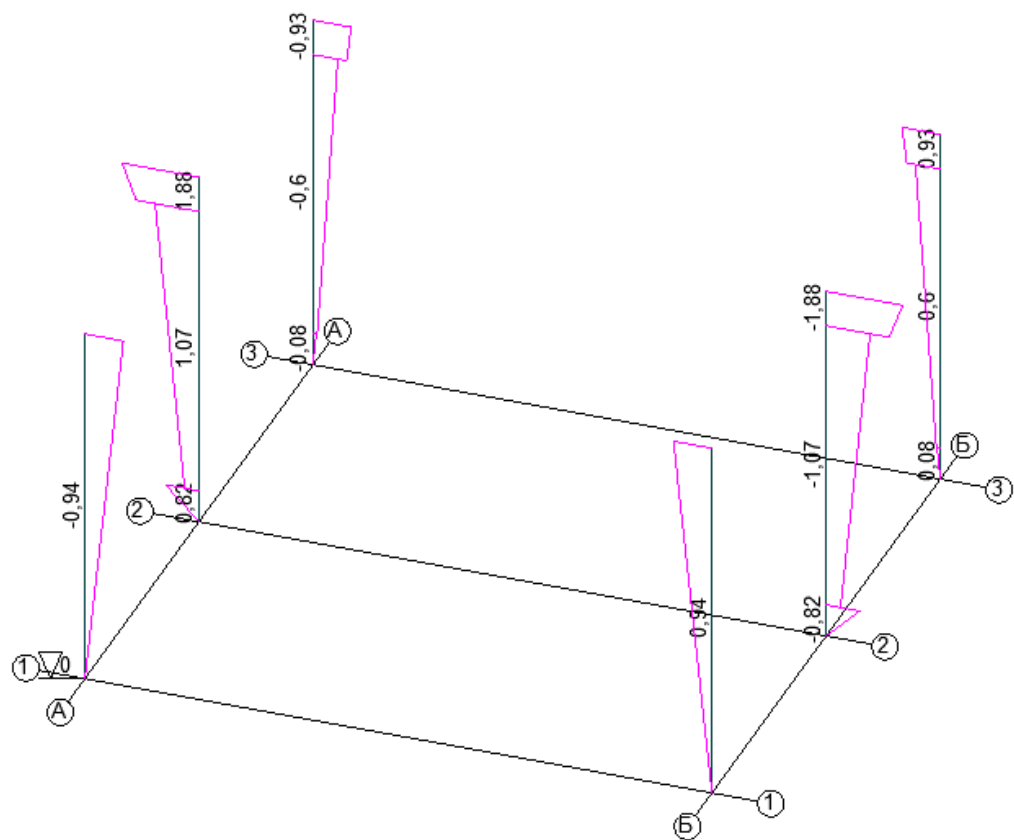
Рисунок 2.9 – Эпюры усилий M_y . Колонны
