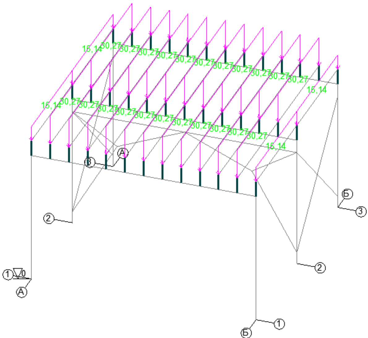
Рисунок 2.3 – Приложенная постоянная нагрузка на второстепенные балки
