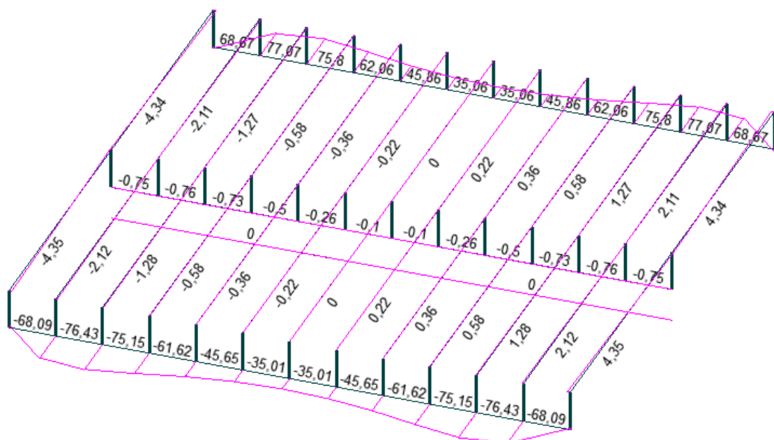
Рисунок 2.7 – Балки перекрытия. Эпюры усилий M_z
