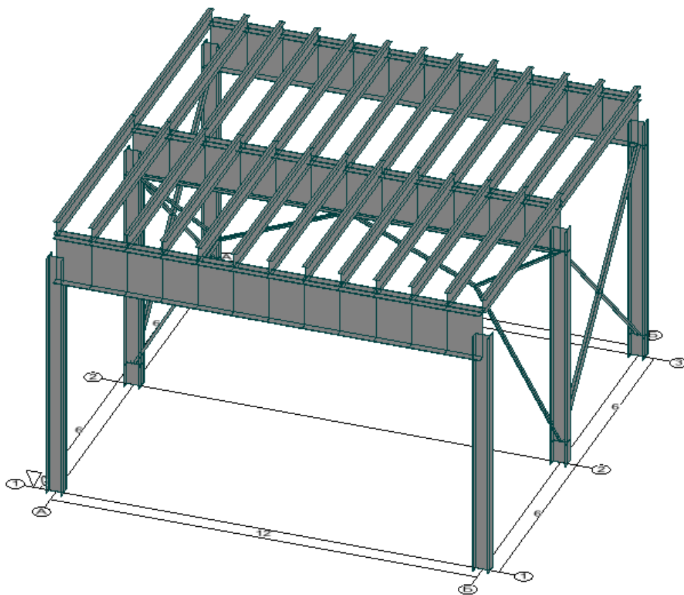
Рисунок 2.1 – Расчетная схема балочной клетки
