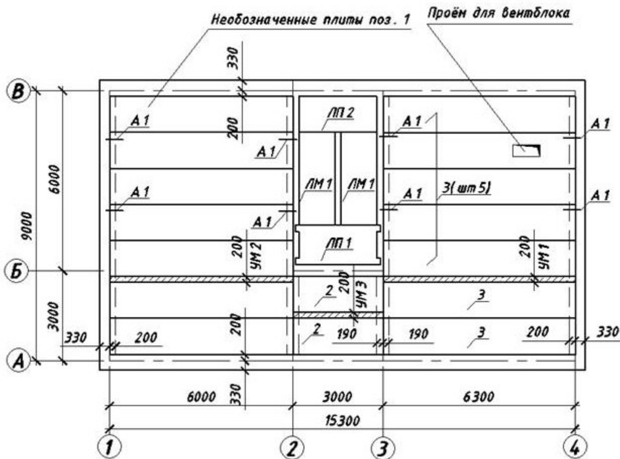
Рисунок 2 – План перекрытий первого этажа малоэтажного дома.
