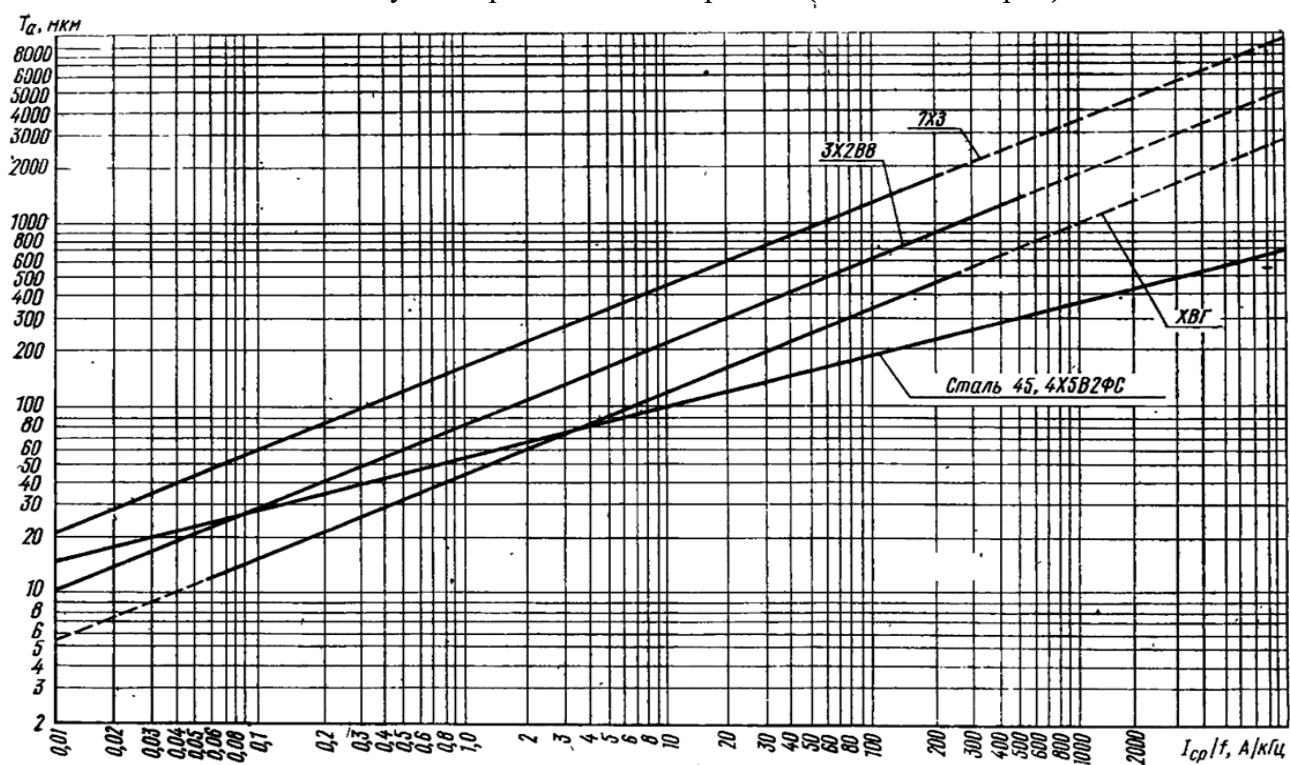
Рисунок 3.3 – Зависимость глубины изменённого слоя от соотношения среднего тока к частоте импульсов (электрод-инструмент – медь)
