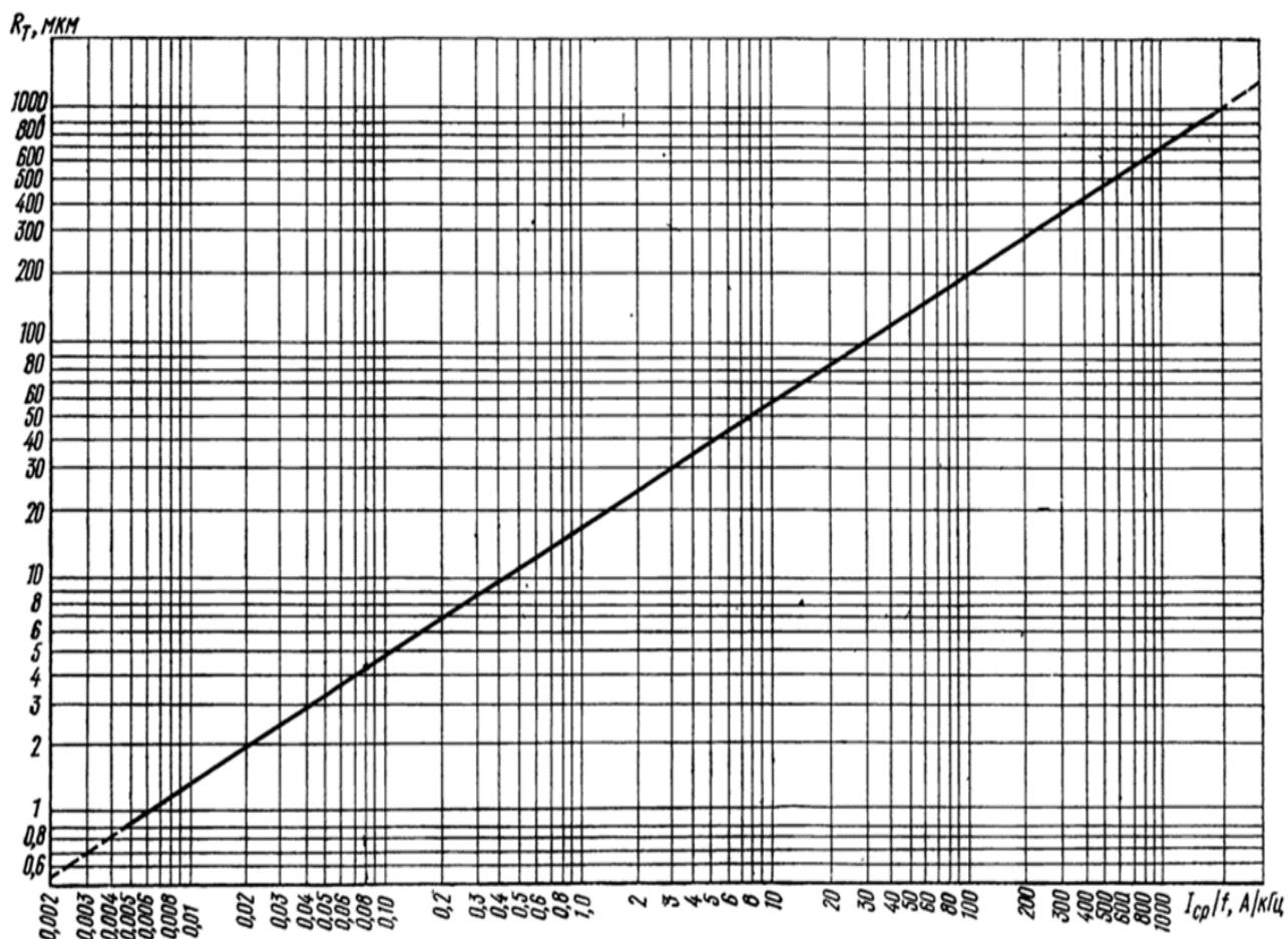
Рисунок 3.2 – Зависимость высоты микронеровностей от соотношения среднего тока к частоте импульсов различных материалов (медный электрод)
