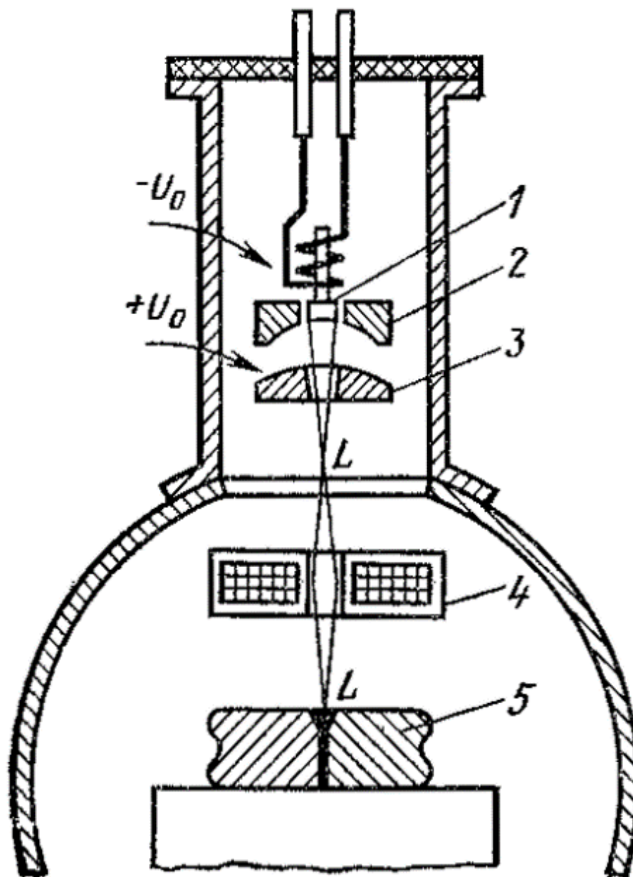
Рисунок 4.1 — Схема электронно-лучевой установки
