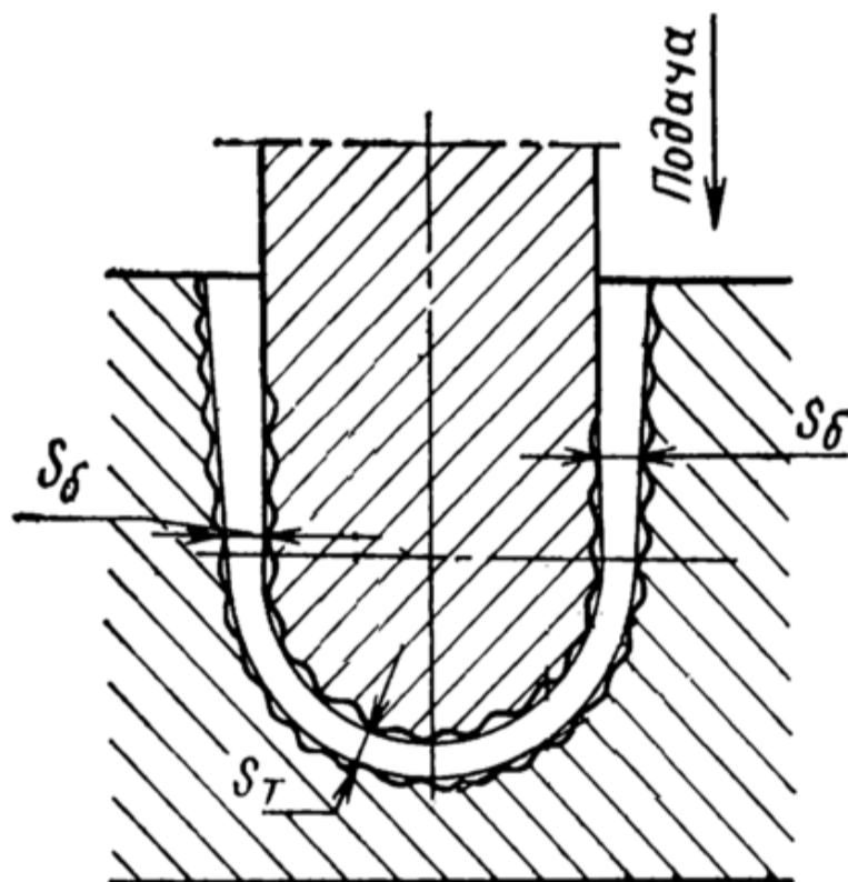
Рисунок 3.1 – Виды межэлектродного зазора при прошивании отверстий
