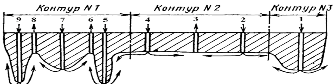
Рисунок 2.1 – Пример контура электрода со схемой циркуляции жидкости
