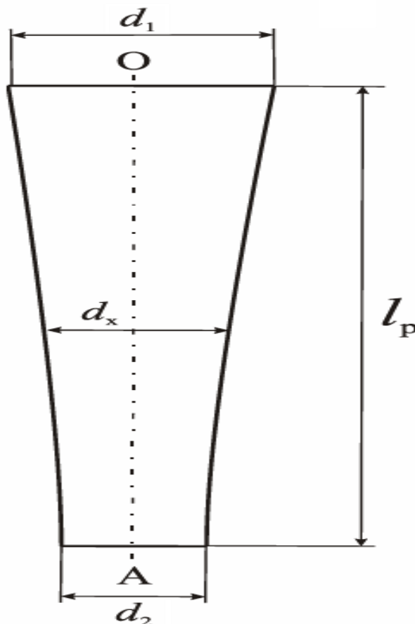
Рисунок 6.1 – Круглый экспоненциальный волновод
