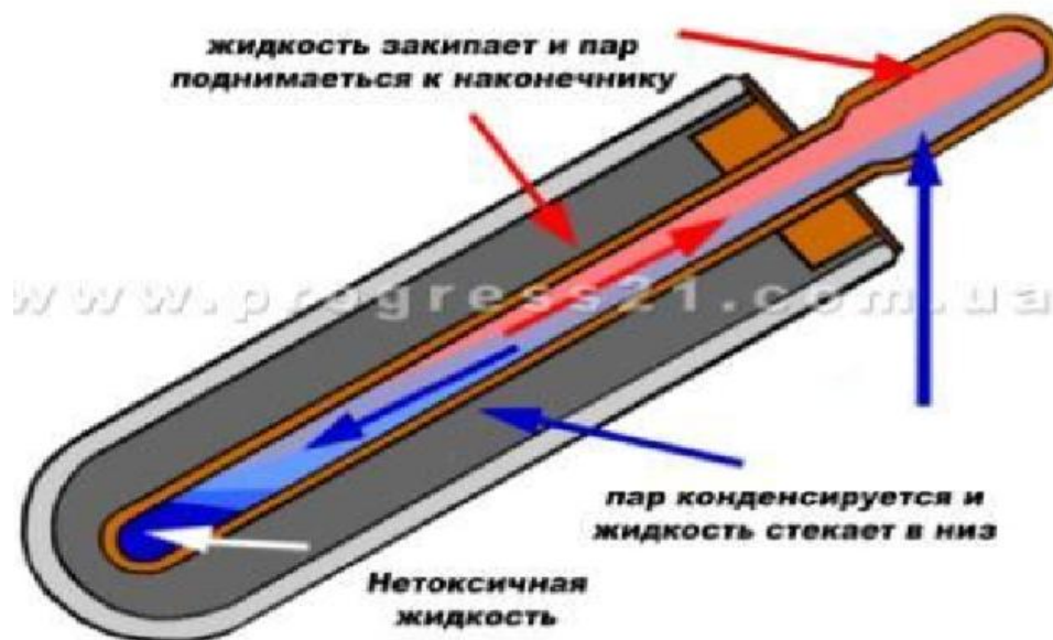
Рисунок 1– Вакуумная трубка
