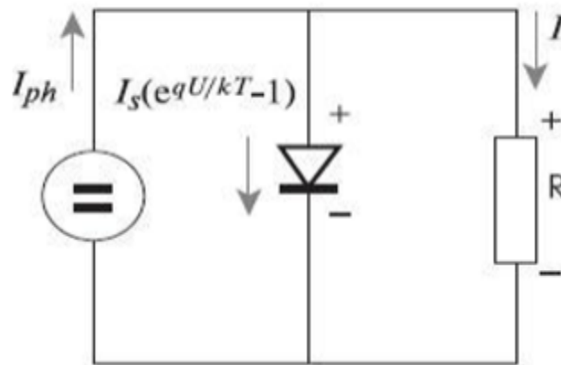
Рисунок 11 – Эквивалентная схема солнечного элемента
