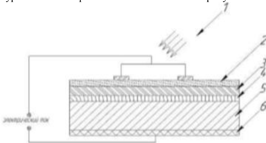
1 – солнечное излучение (фотоны); 2 – наружный контакт; 3 – отрицательно заряженный слой; 4 – слой утечки; 5 – положительно заряженный слой; 6 – внутренний контакт Рисунок 10 – Структура полупроводникового фотоэлемента
